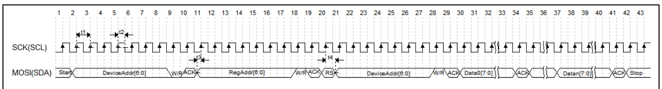
图 9-8 I2C 读时序
